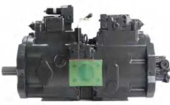
K5V160DTP-9Y04-13T( SH350A)
